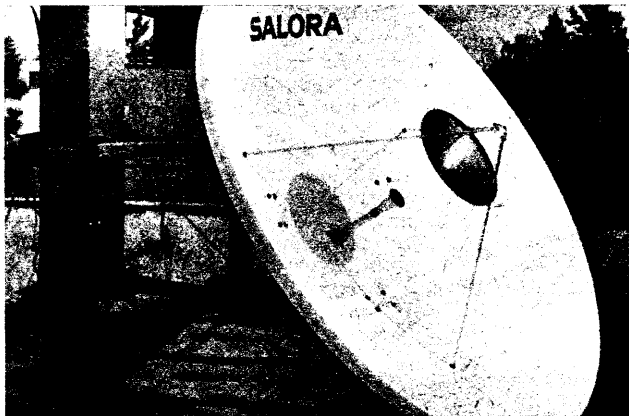
Obr. 14. Umístění antény typu Cassegrain o průměru 180 cm na betonovém sloupku, který je součástí střešní konstrukce
